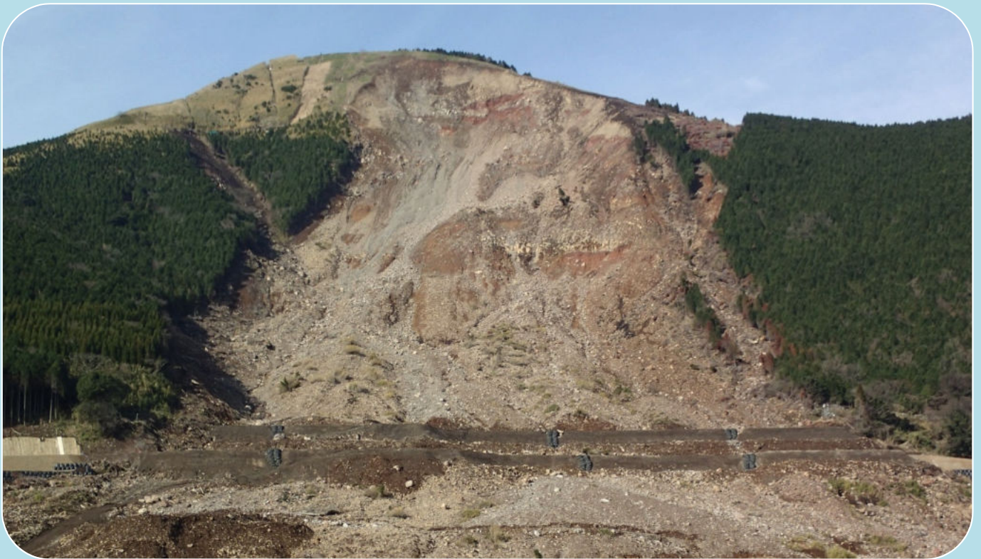
阿蘇大橋地区斜面崩壊対策の進捗状況 (平成28年12月24日撮影)
