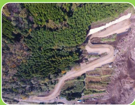
1号工事用道路ドローン撮影状況 □ 崩壊斜面へのアクセス用（工事用道路）を施工しています □
